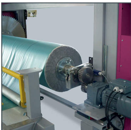
Motorbetriebene PVB/EVA-Abrollvorrichtung
