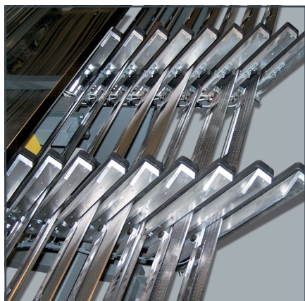
Магазин для хранения до 15 различных типов профиля
