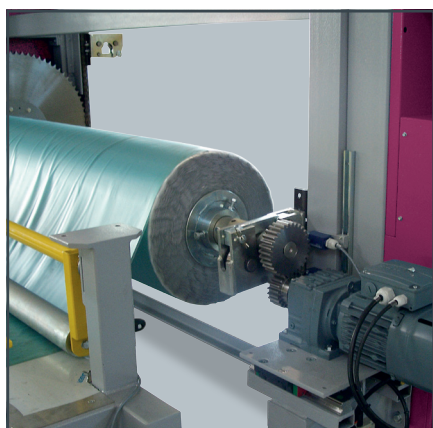
Приводное устройство для разматывания PVB/EVA
